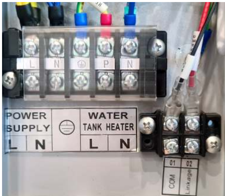
Obrázok 11: Elektrické zapojenie kabeláže vo vnútri vnútornej jednotky tepelného čerpadla
