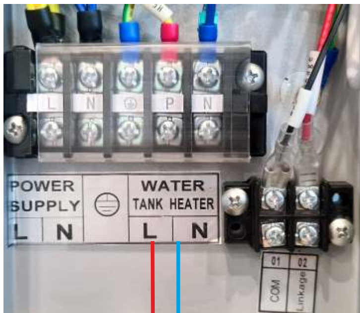
Obrázok 8: Elektrické zapojenie kabeláže vo vnútri vnútornej jednotky tepelného čerpadla
