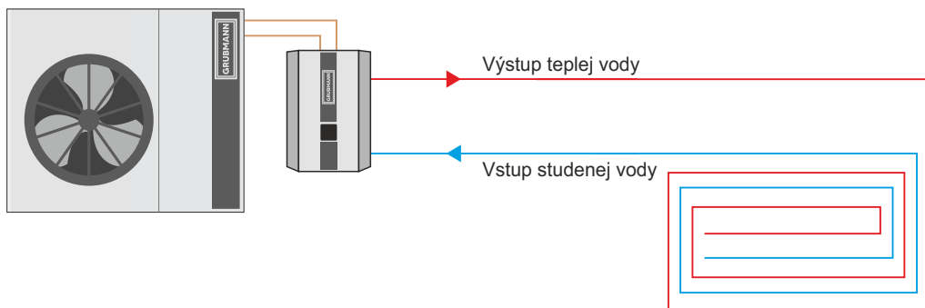
Obrázok 10: Systémová schéma zapojenia
