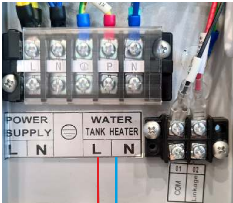
Obrázok 6: Elektrické zapojenie kabeláže vo vnútri vnútornej jednotky tepelného čerpadla
